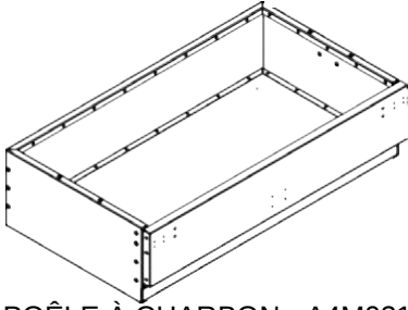
C01 POÊLE À CHARBON - A4M02135 (x1) 1 15/16"x25 1/4"x44 13/16" (292x642x1139)
