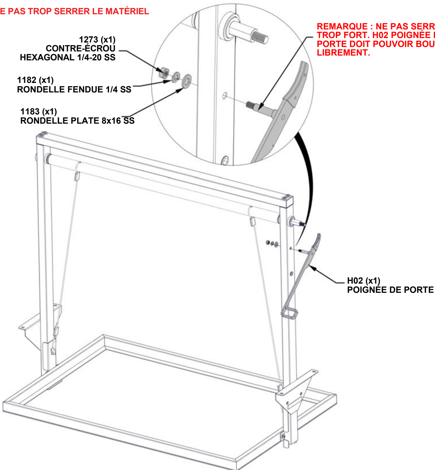
H02 POIGNÉE DE PORTE - A4M02497 (x1) 7/8"x3 5/8"x11 1/4" (22x92x285)
