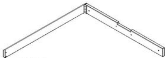
WP8 (x2) | ASSEMBLAGE DU LINTEAU - W2A01926
