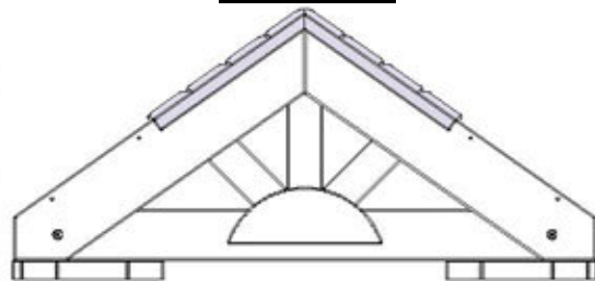
ASSEMBLAGE CORRECT DE PANNEAU DE TOIT
