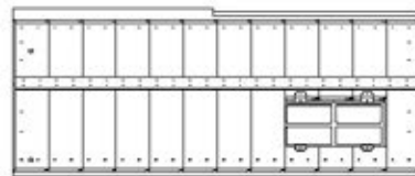
WP2 (x1) | PANNEAU DE COIN ARRIÈRE DROIT - W2A03490
